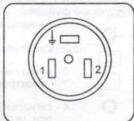
Условная маркировка контактов розетки
